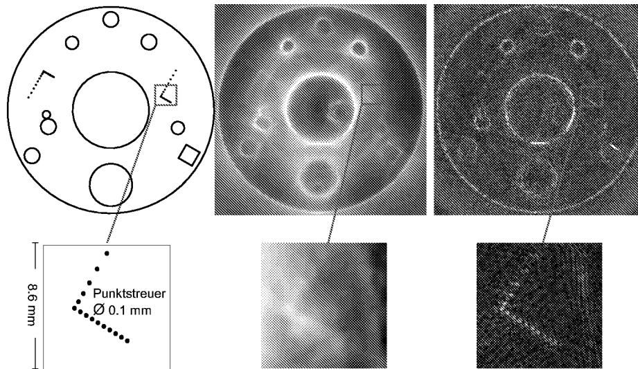
Abb. 1. Ultraschall-Phantom und rekonstruierte Bilder. Links: Skizze des Ultraschallphantoms mit Ausschnittsvergrößerung. Der Durchmesser des Phantoms beträgt 8.5 mm. Die kleinsten Strukturen sind Nylonfäden mit einem Durchmesser von jeweils 0.1 mm und einem Abstand von 0.5 mm. Mitte: USCT-Bildrekonstruktion unter Verwendung der Amplitudeninformationen der aufgenommenen Ultraschallsignale. Rechts: USCT-Bildrekonstruktion unter Verwendung der Amplituden- und Phaseninformationen. Die Nylonfäden können klar trennbar abgebildet werden.
