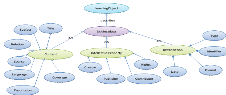
Fig. 4. Ontología DCOntoRep
