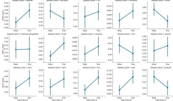
FIGURE 4 – Comparaison des performances des modèles avec ou sans instruction sur l'ensemble des données.
