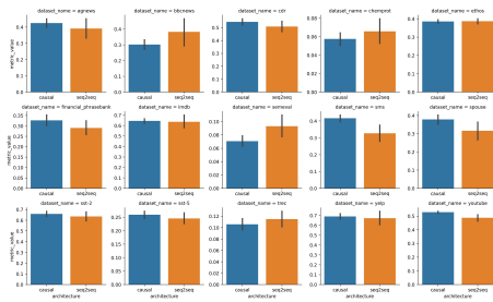
FIGURE 2 – Variation des performances entre les différentes architectures.
