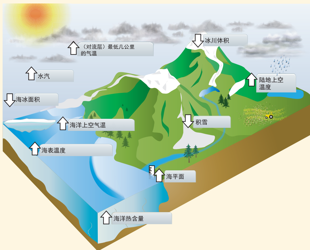
常见问题2.1, 图1 | 对将随全球变暖发生变化的气候系统众多组分的独立分析显示出与变暖相一致的趋势(箭头方向表示变化的符号), 如FAQ2.1, 图2所示。
