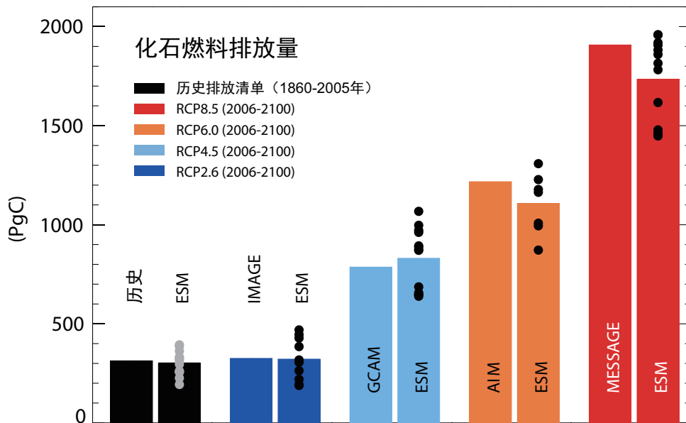
图TS.19 | 在所有四个RCP情景下，由各CMIP5模式模拟的可兼容的化石燃料排放量。(上图) 年排放的时间序列 (PgC/年)。虚线表示历史估值和可用于确定RCP情景的若干综合评估模式 (IAM) 计算的RCP排放量。实线和羽状轮廓表示各CMIP5地球系统模式结果 (ESM，模式均值，阴影区内为1个标准差)。(下图) 针对历史估值和RCP情景模拟的历史时期 (1860-2005年) 和21世纪 (在CMIP5中定义为2006-2100年间) 的累计排放量。左侧直方表示各IAM模式给出的累计排放量，右侧直方表示各CMIP5 ESM给出的多模式平均估值，而点线表示各单个ESM结果。从各CMIP5 ESM结果中看出，可跟踪陆地-大气-海洋系统的碳总量，而该碳总量的变化必须等于排入该系统的化石燃料排放量。因此，通过以下等式给出兼容的排放量：累计排放量 = \Delta C_A + \Delta C_L + \Delta C_O ，而排放率 = d/dt [C_A + C_L + C_O] ，式中 C_A ， C_L ， C_O 分别为存留在大气、陆地和海洋中的碳。此图没有考虑百年时间尺度上很小的其它CO 2 源和汇，如火山、沉积或岩石风化等。{文框6.4；图6.25}
