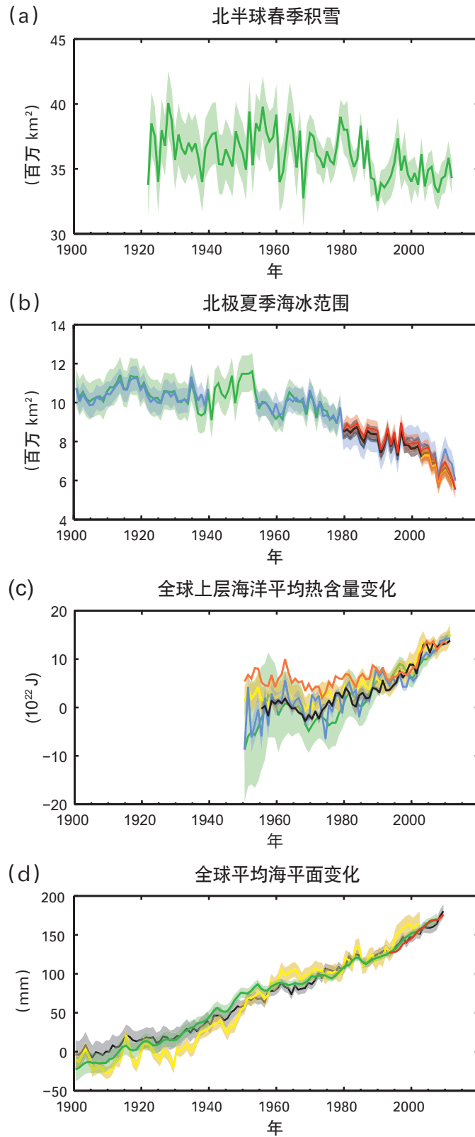
图SPM.3 | 观测到的多项全球气候变化指标：(a) 北半球3-4月（春季）平均积雪范围；(b) 北极7-8-9月（夏季）平均海冰范围；(c) 调整到2006-2010年时段相对于1970年所有资料集平均值的全球平均海洋上层（0 - 700m）热含量变化；(d) 相对于1900-1905年最长的连续资料集平均值的全球平均海平面，所有资料集均调整为1993年（即有卫星高度仪资料的第一年）的相同值。所有时间序列（不同颜色的曲线表示不同的资料集）给出年度值，经评估后的不确定性用不同颜色的阴影区表示。关于资料集列表，见技术摘要的补充材料{图3.2, 图3.13, 图4.19和图4.3；常见问题2.1, 图2；图TS.1}
