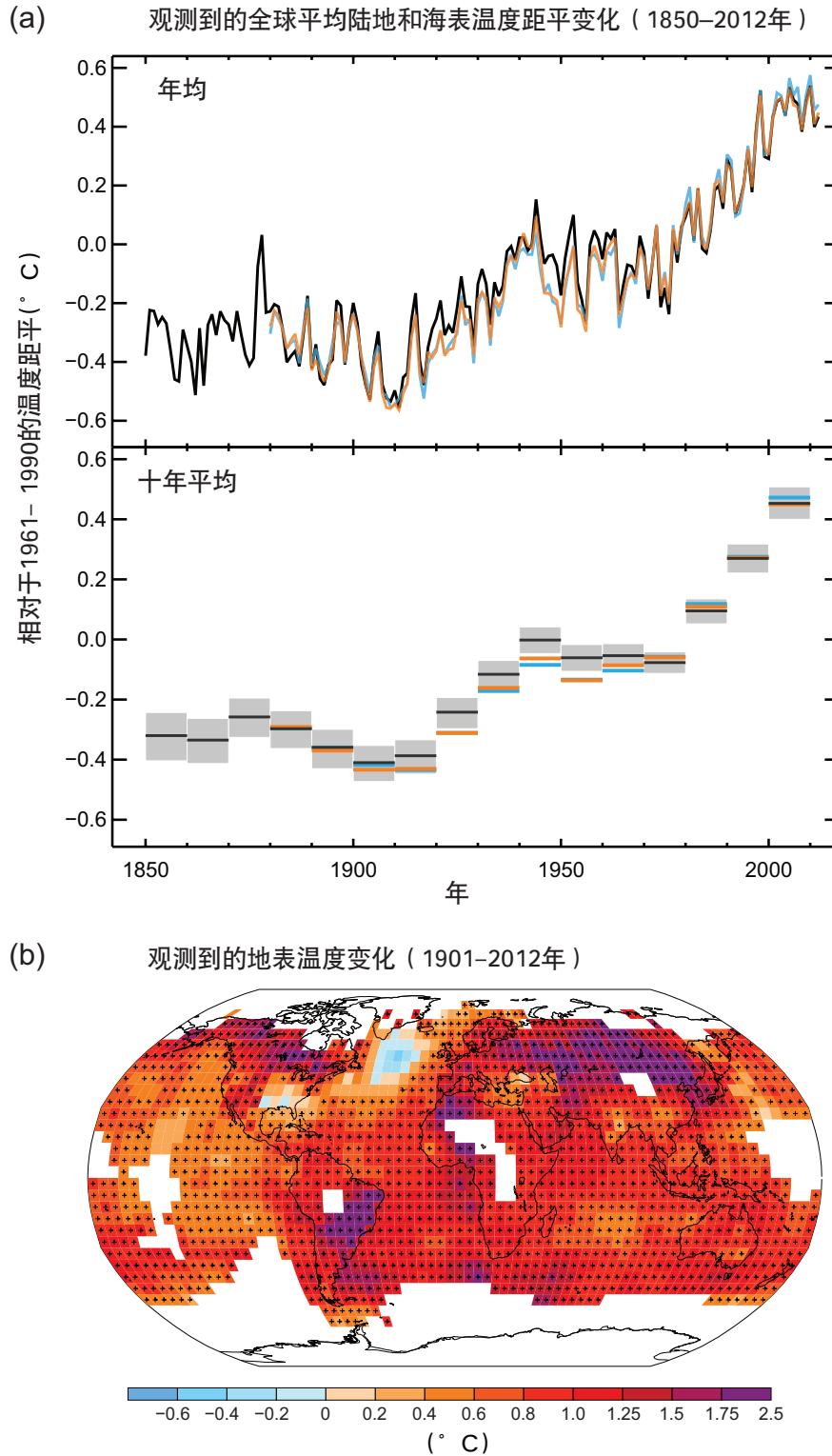
图SPM.1 | (a) 观测到的全球平均陆地和海表温度距平(1850–2012年)，源自三个资料集。上图：年均值，下图：十年均值，包括一个资料集(黑色)的不确定性估计值。各距平均相对于1961–1990年均值。(b) 观测到的地表温度变化(1901–2012年)，温度变化值是通过对其趋势进行了线性回归所确定的趋势计算得出的。只要可用资料能够得出确凿估算值，均对其趋势作了计算(即仅限于该时期前10%和后10%时段内，观测记录完整率超过70%并且资料可用率大于20%的格点)，其它地区为白色。凡是趋势达到10%显著性的格点均用“+”号表示。有关资料集清单和更多技术细节，详见技术摘要的补充材料{图2.19–2.21；图TS.2}
