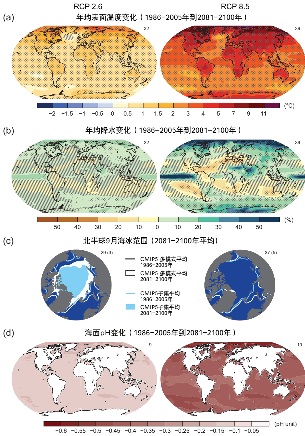
图SPM.8 | CMIP5多模式在RCP2.6和RCP8.5情景下对2081-2100年模拟的平均结果：(a) 年均表面温度变化，(b) 年均降水百分率变化，(c) 北半球9月海冰范围，以及(d) 海洋表面pH的变化。图(a)、(b)和(d)部分的变化相对于1986-2005年。每个部分右上角都标明了用于计算多模式平均的CMIP5模式数量。图(a)和(b)中的阴影是指多模式平均值小于内部变率的地区（即，小于20年平均自然内部变率一个标准差）。点状部分是指多模式平均值大于自然内部变率（即，大于20年平均自然内部变率两个标准差）且90%的模式在变化特征上吻合的地区（见文框12.1）。图(c)中，线条表示模拟的1986-2005年均值；填充部分是本世纪末的均值。白色是CMIP5的多模式平均值，浅蓝色是最准确重现北极气候平均状况和北极海冰范围1979-2012年趋势的模式子集（模式的数量见括号）预估的平均海冰范围。更多的技术细节参见技术摘要补充材料。（图6.28，12.11，12.22和12.29；图TS.15，TS.16，TS.17和TS.20）
