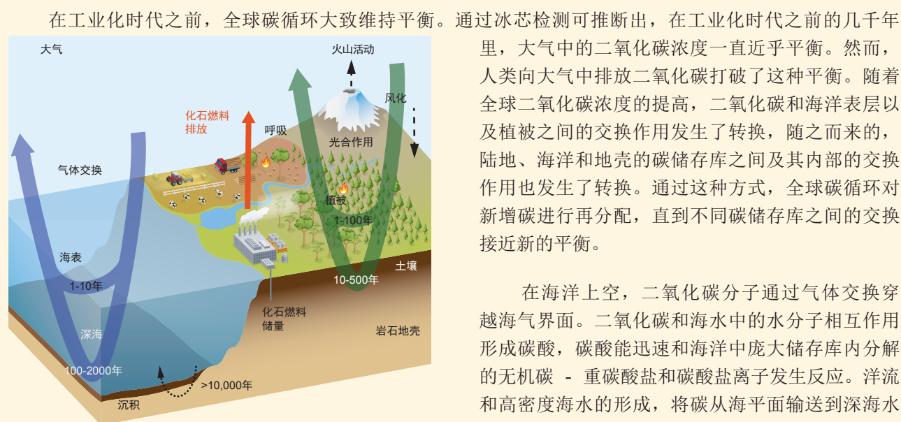
常见问题6.2，图1 | 全球碳循环简图，显示通过主要储存库碳转移的典型周转时间尺度。
