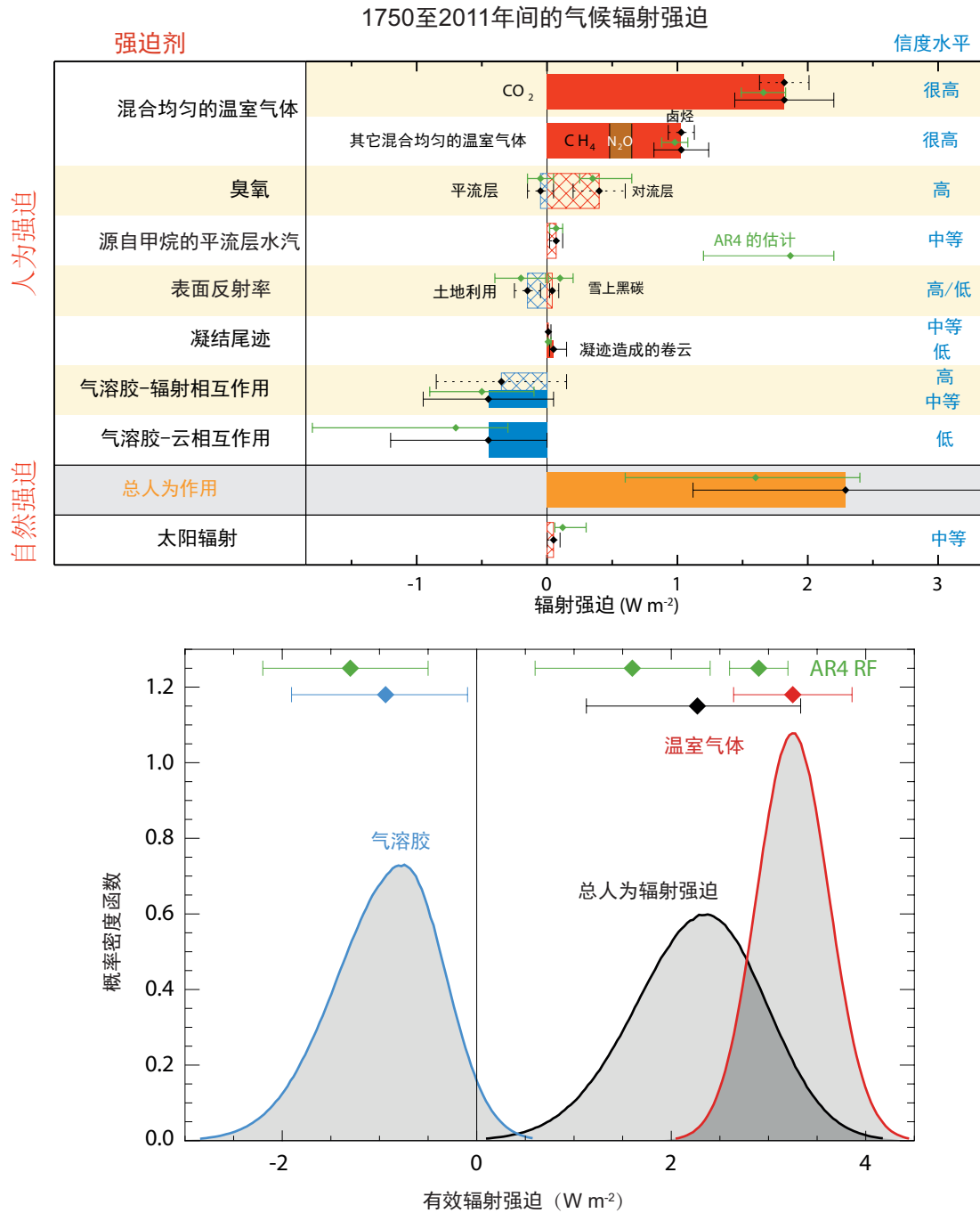
图TS.6 | 工业化时代气候变化的辐射强迫(RF)和有效辐射强迫(ERF)。(上图) 1750-2011年间浓度变化产生的强迫以及相关的不确定性区间(实心直方为有效辐射强迫, 阴影直方为辐射强迫, 绿菱形和相关不确定性是指AR4评估的辐射强迫)。(下图) 气溶胶和温室气体(GHG)的有效辐射强迫以及总有效辐射强迫的概率密度函数(PDF)。绿线表示AR4 辐射强迫90%信度区间, 可与红、蓝及黑线进行对比, 红、蓝及黑线表示AR5有效辐射强迫90%信度区间(尽管辐射强迫和有效辐射强迫有差异, 尤其是对于气溶胶)。地表反照率变化和组合凝结尾流以及凝结尾流卷云等产生的有效辐射强迫已被纳入总人为强迫, 但并未被列为单独的概率密度函数。对于某些强迫机制(臭氧、土地利用、太阳), 辐射强迫假定为代表有效辐射强迫, 但额外17%的不确定性以正交添加到辐射强迫的不确定性。{图8.15, 8.16}
